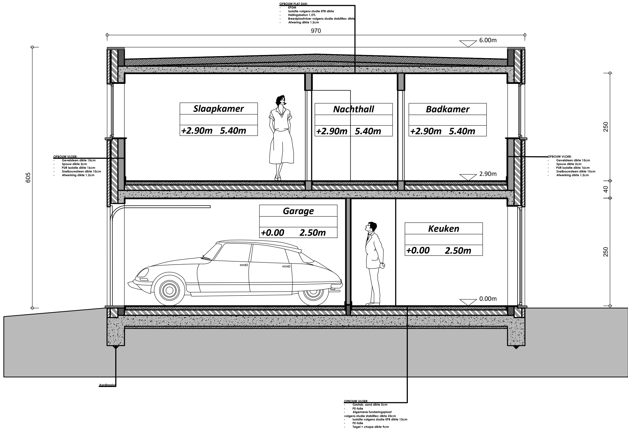
SNEDE A-A'
